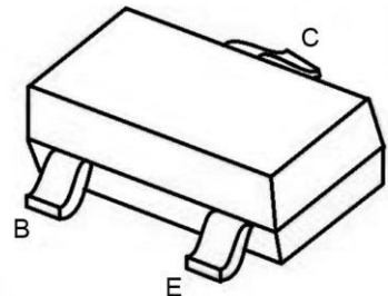
SOT-23
